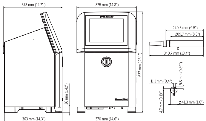
Las dimensiones mostradas se corresponden con el modelo IP66
